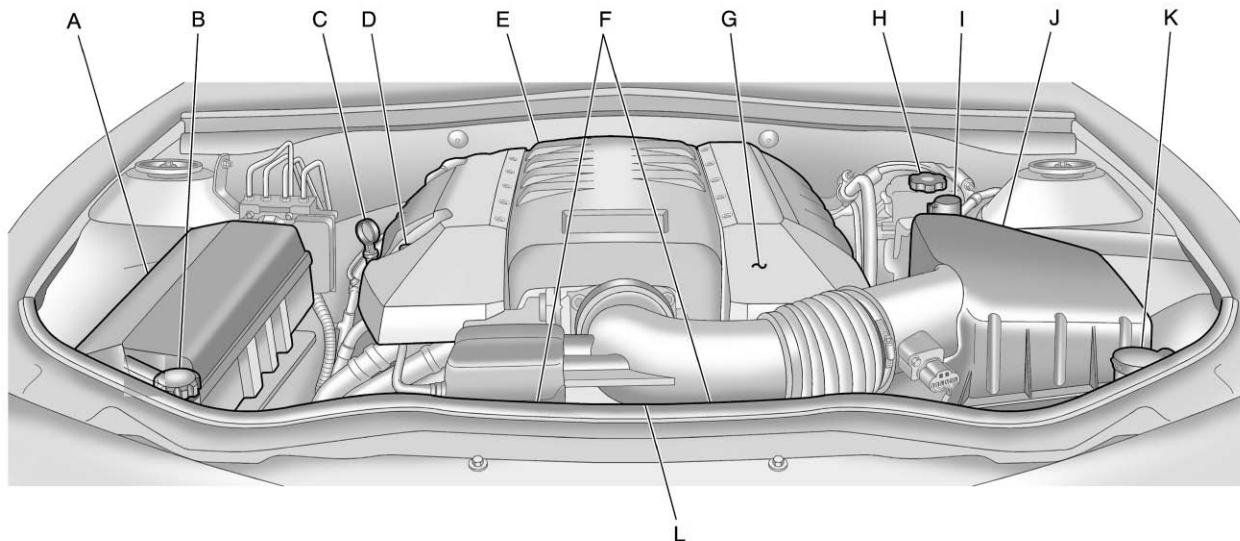
Moteur V8 6.2L (moteur L99 illustré, LS3 similaire)
