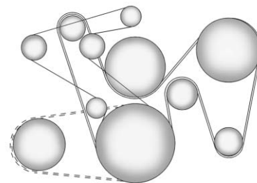
Moteurs V8 6.2L (LSA)
