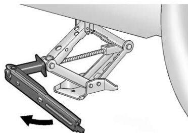
Cric à tête hexagonale et clé
